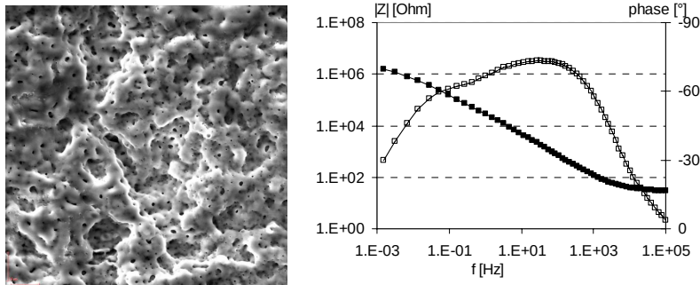
Abbildungen: REM SE Bild (links), EIS-Diagramm (rechts)
